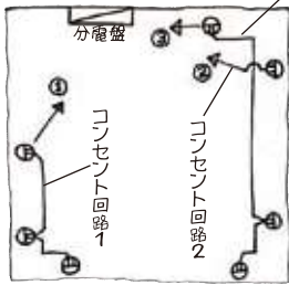
コンセント回路図
